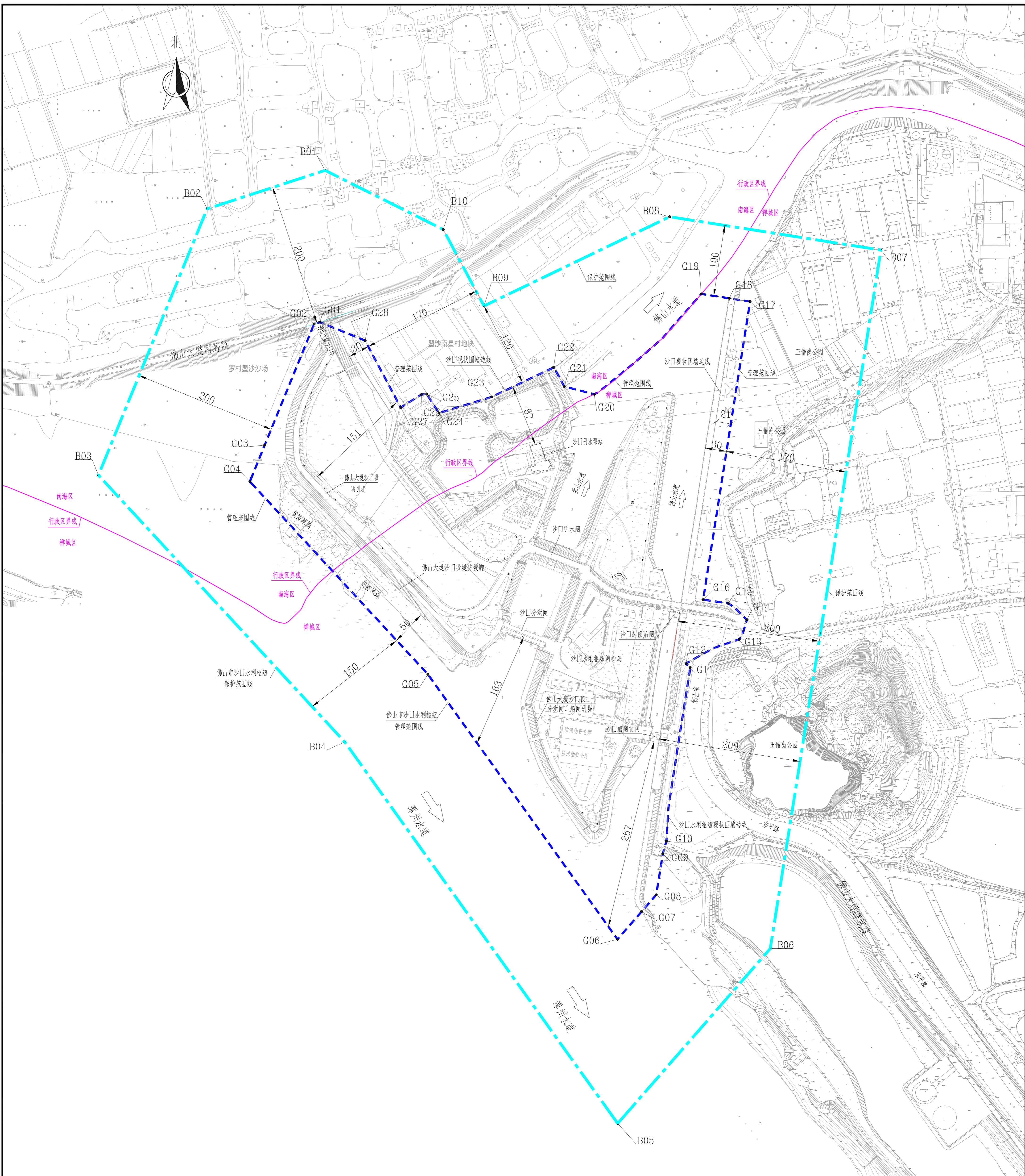
佛山市沙口水利枢纽管理和保护范围平面布置图 1:2500
